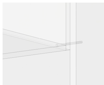
Compact HPL sienelės tvirtinimas po stalviršiu
